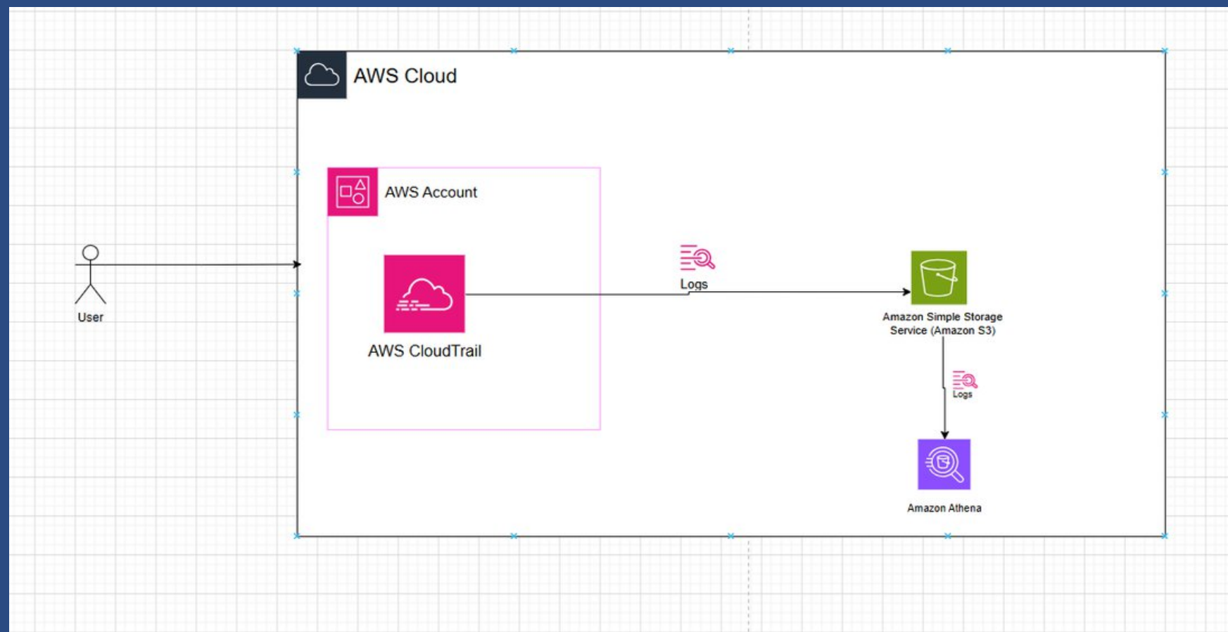
Sơ đồ Luồng dữ liệu Logs
